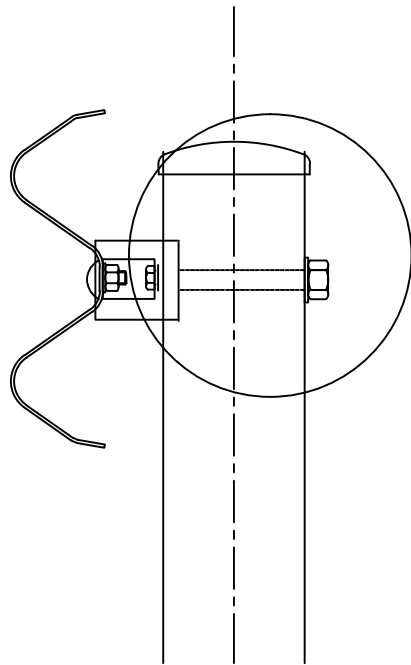
托架大样图1:10
