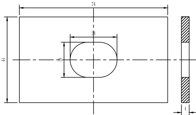
横梁垫片 1:1
