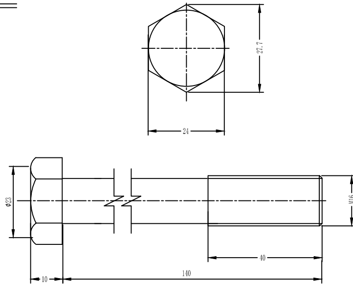
连接螺栓大样图 1:1
