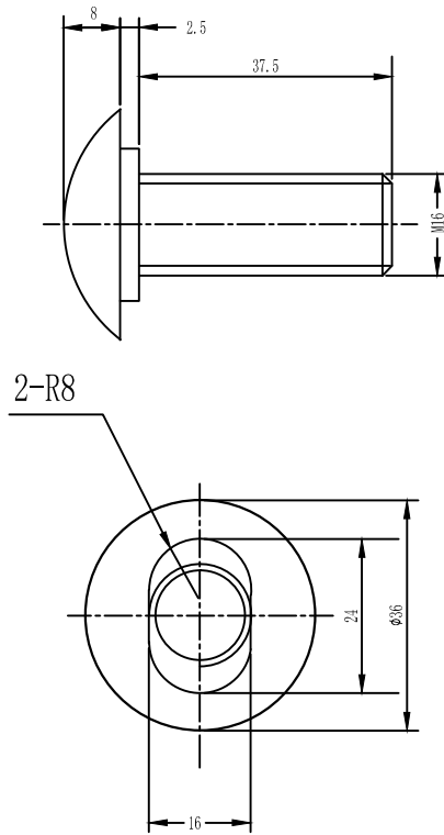
拼接螺栓大样图 1:0.75
