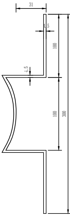
托架立面图1:5
